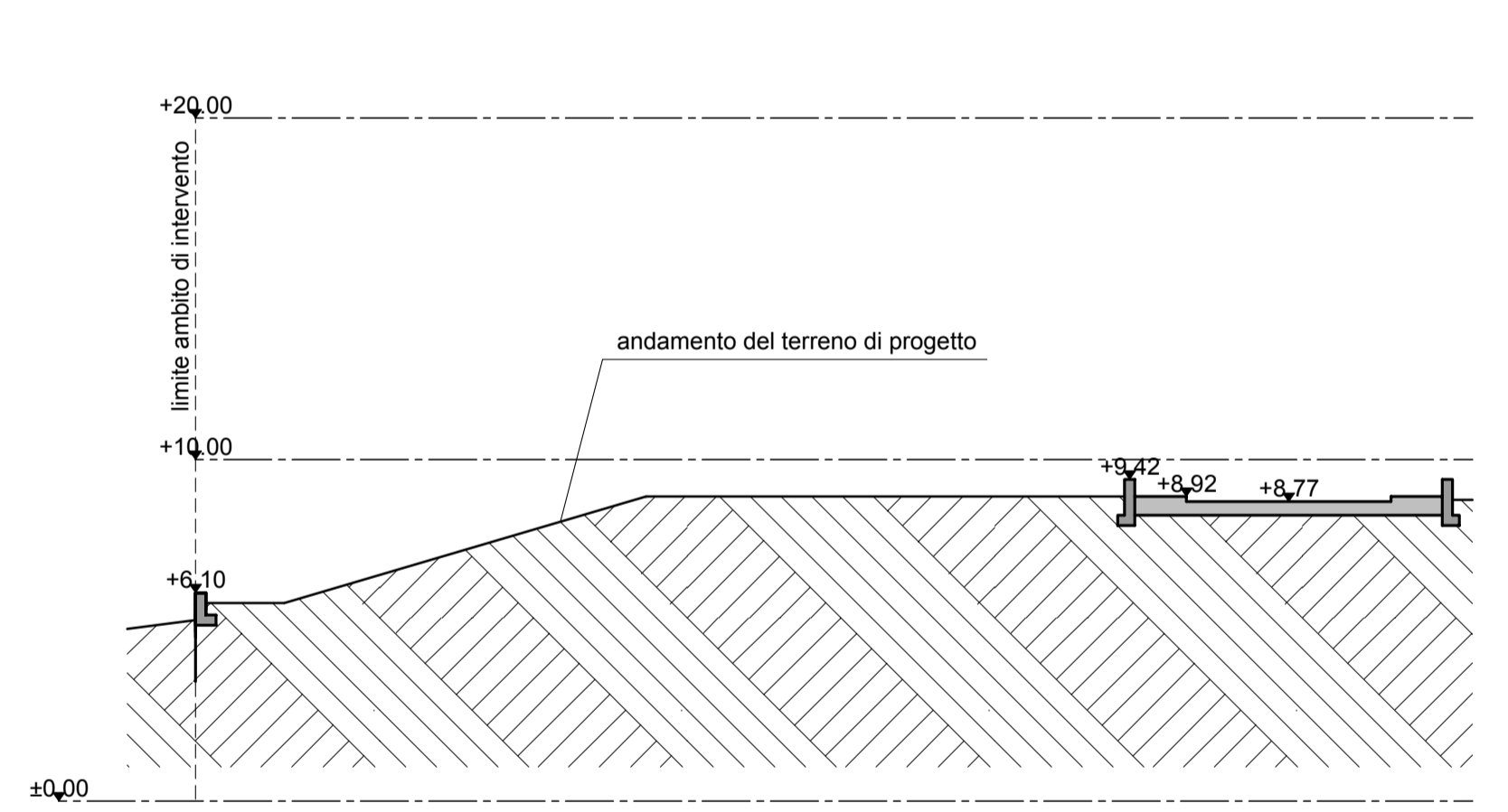
Sezione D-D - scala 1/200
