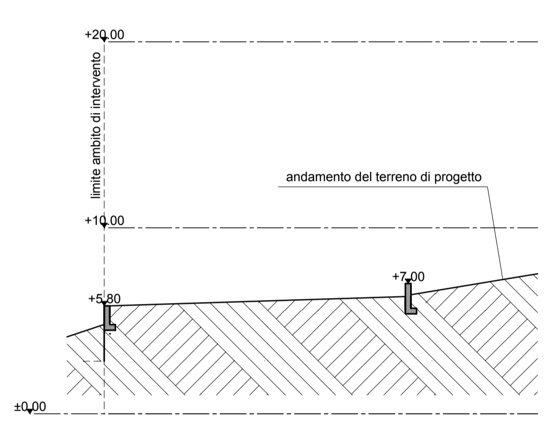
Sezione B1-B1 - scala 1/200
