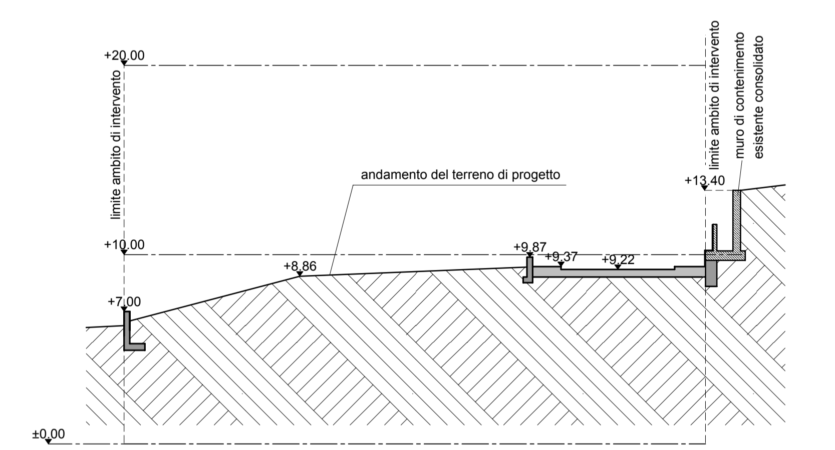
Sezione C-C - scala 1/200
