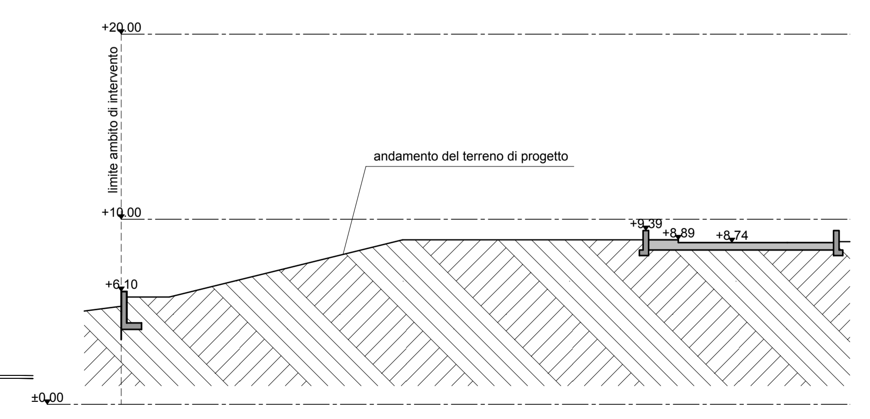
Sezione E-E - scala 1/200
